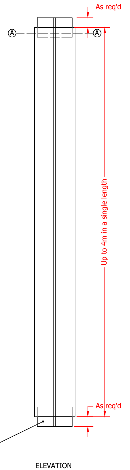
ELEVATION
