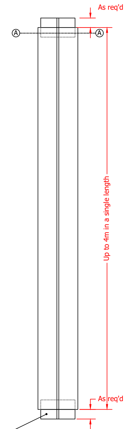
ELEVATION
