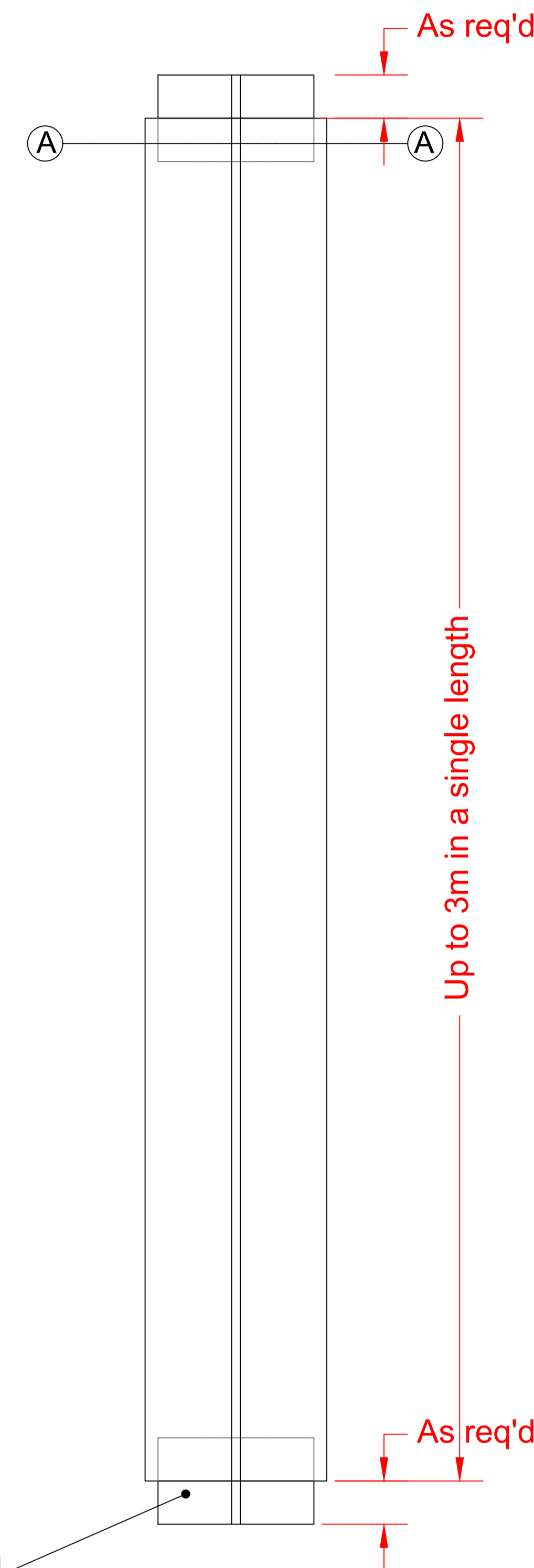
ELEVATION
